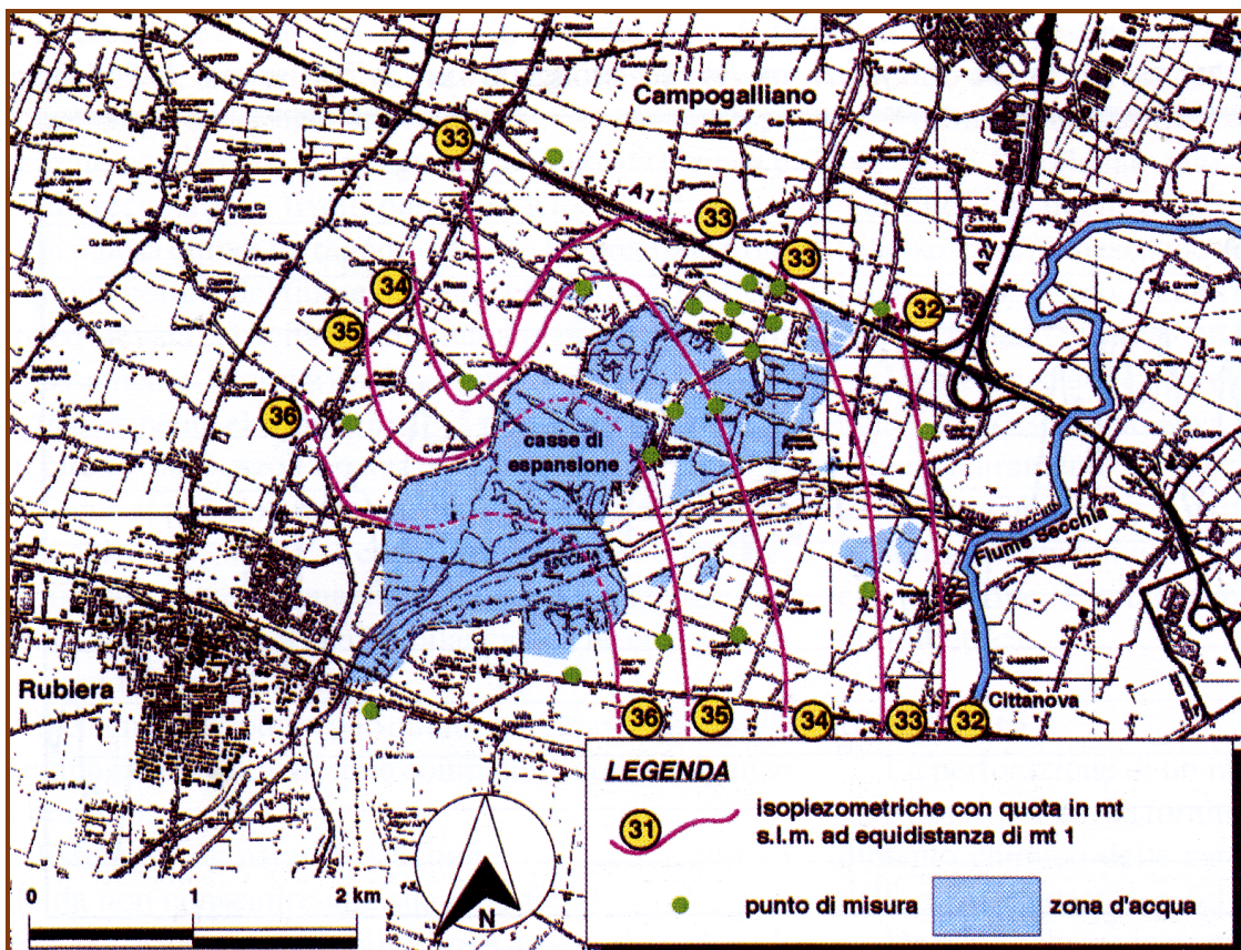
Figura 32 – Isopezometriche delle falde dei conoidi "recente" e "sepolto" – Novembre 1991 2 .
