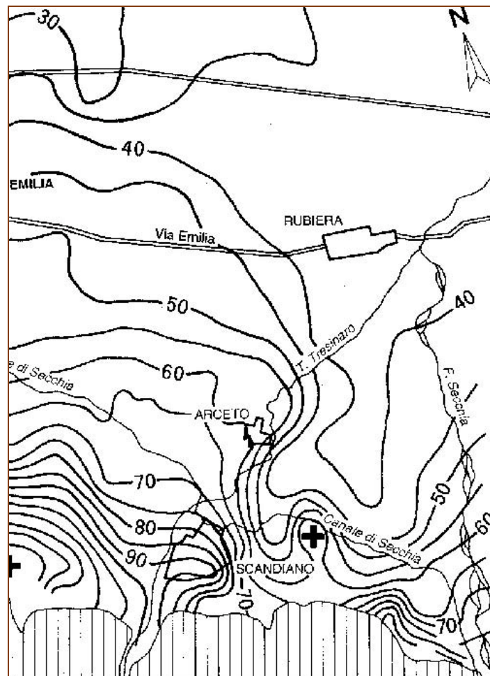
Figura 11 – Isopiezometriche relative al 1991 – Dati AGAC.
