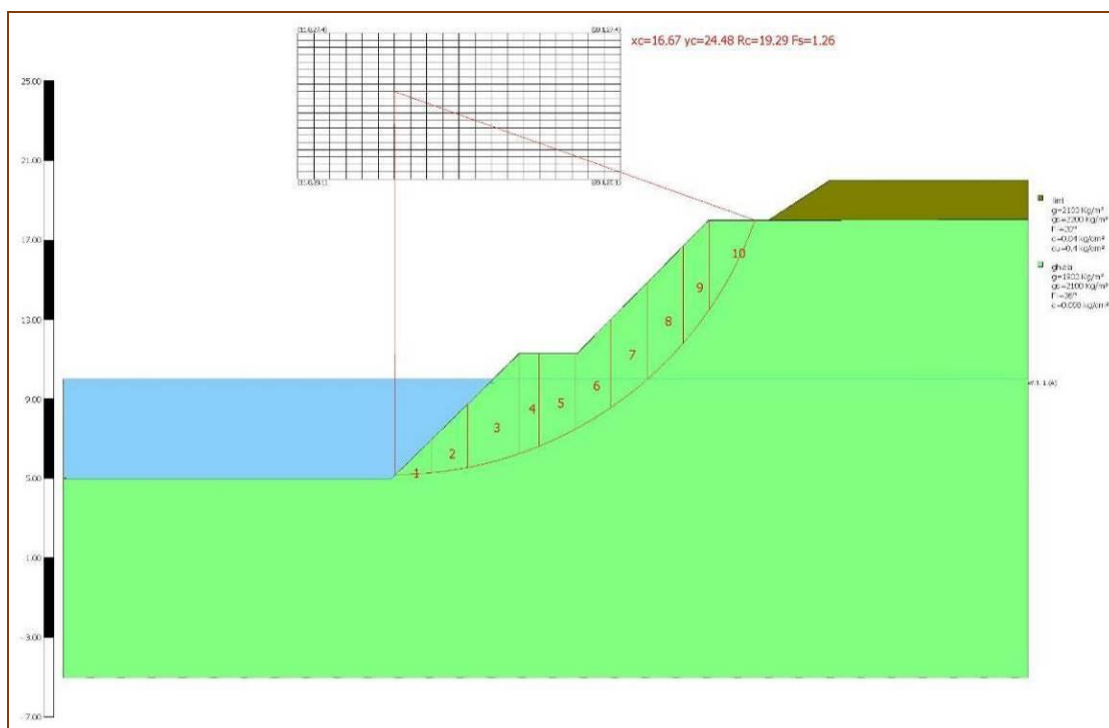
Figura 45 – Calcolo stabilità scarpata di scavo in condizioni statiche.
