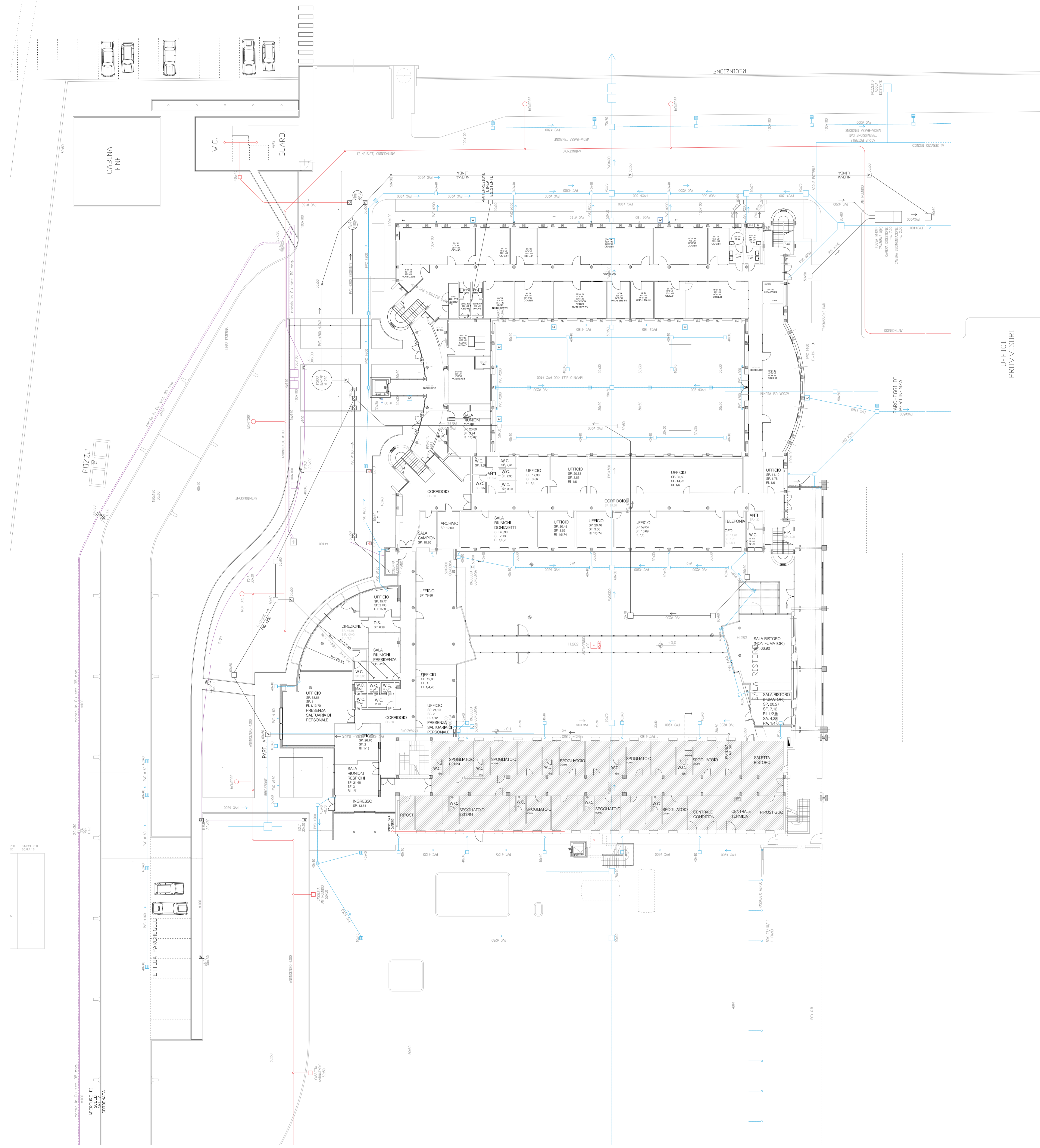
SCHEMA SISTEMA FOGNARIO_ scala 1:200
