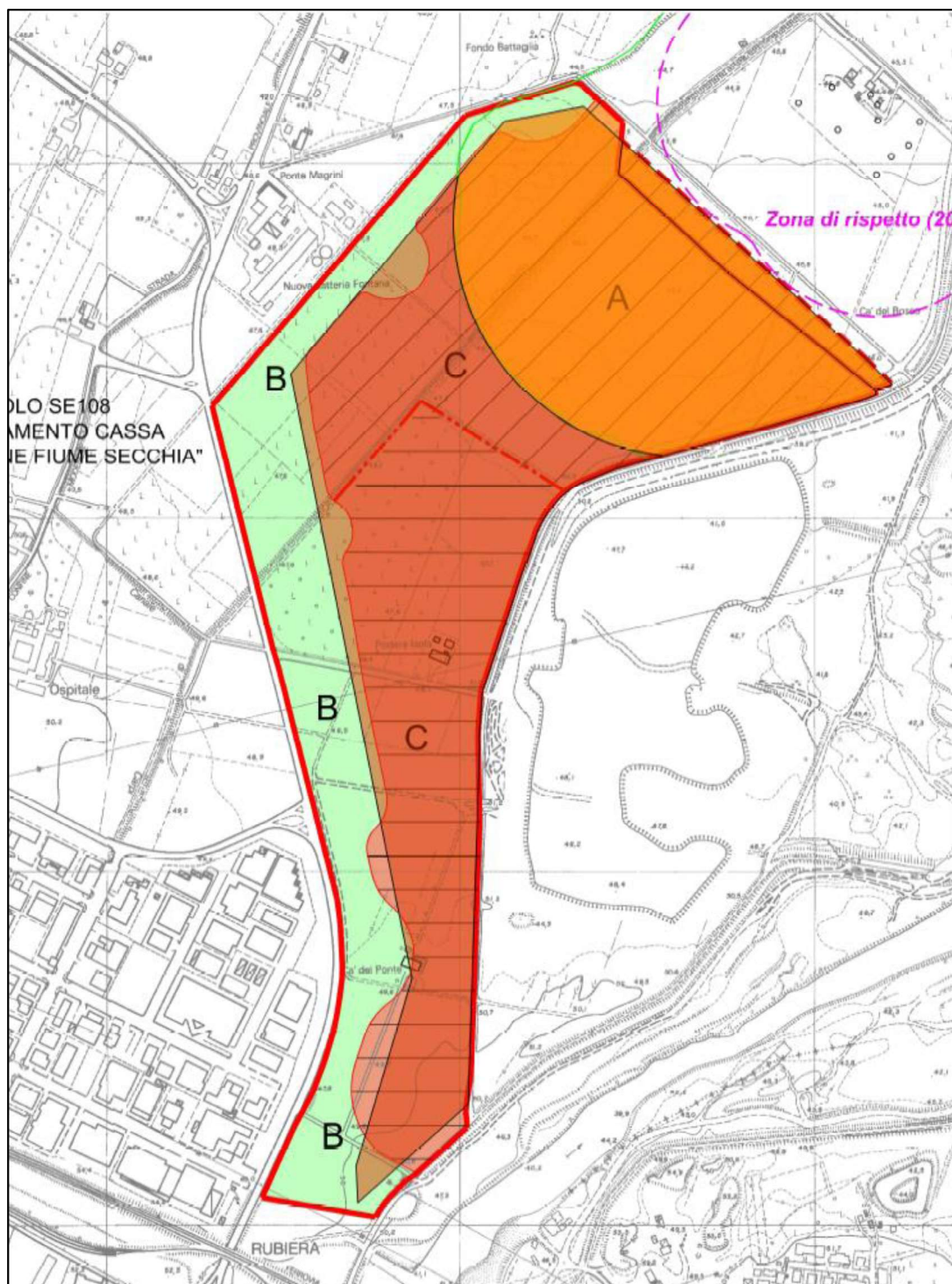
Figura: Sintesi degli interventi di modifica arginatura polo SE108
