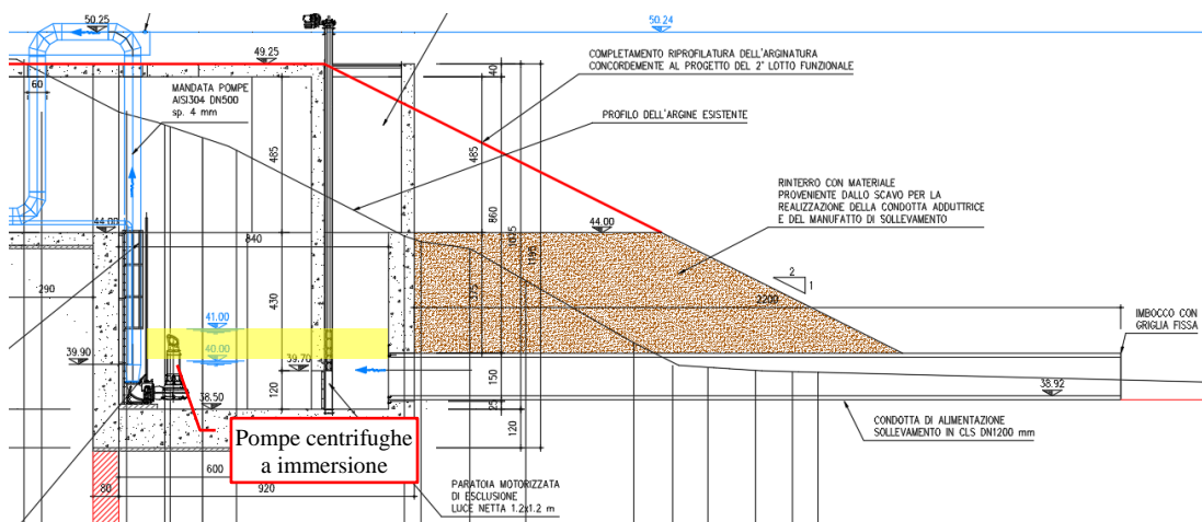
Figura 104. Estratto della sezione di progetto: le pompe lavoreranno sul volume idrico presente tra i 40 e 41 m s.l.m. (fascia colorata in giallo)
