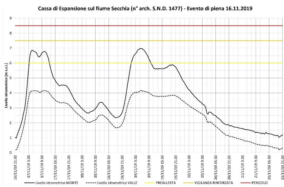
Figura 55. Grafico relativo all'evento di piena del 16 novembre 2019
