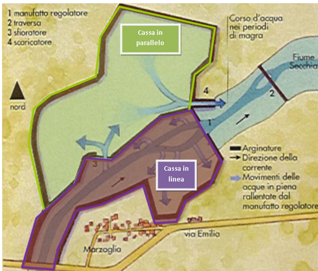
Figura 46. Schema del funzionamento della cassa di espansione
