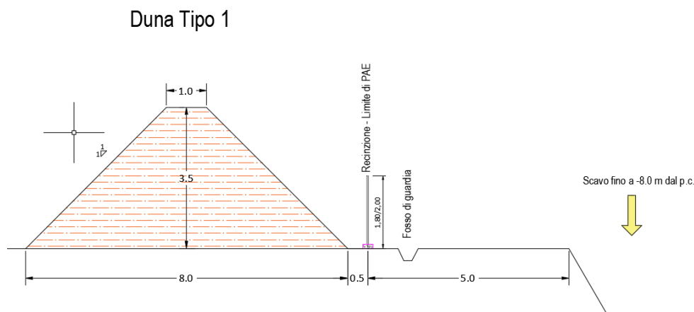
Figura 2. Tipologico della duna posta all'esterno dell'area di PAE
