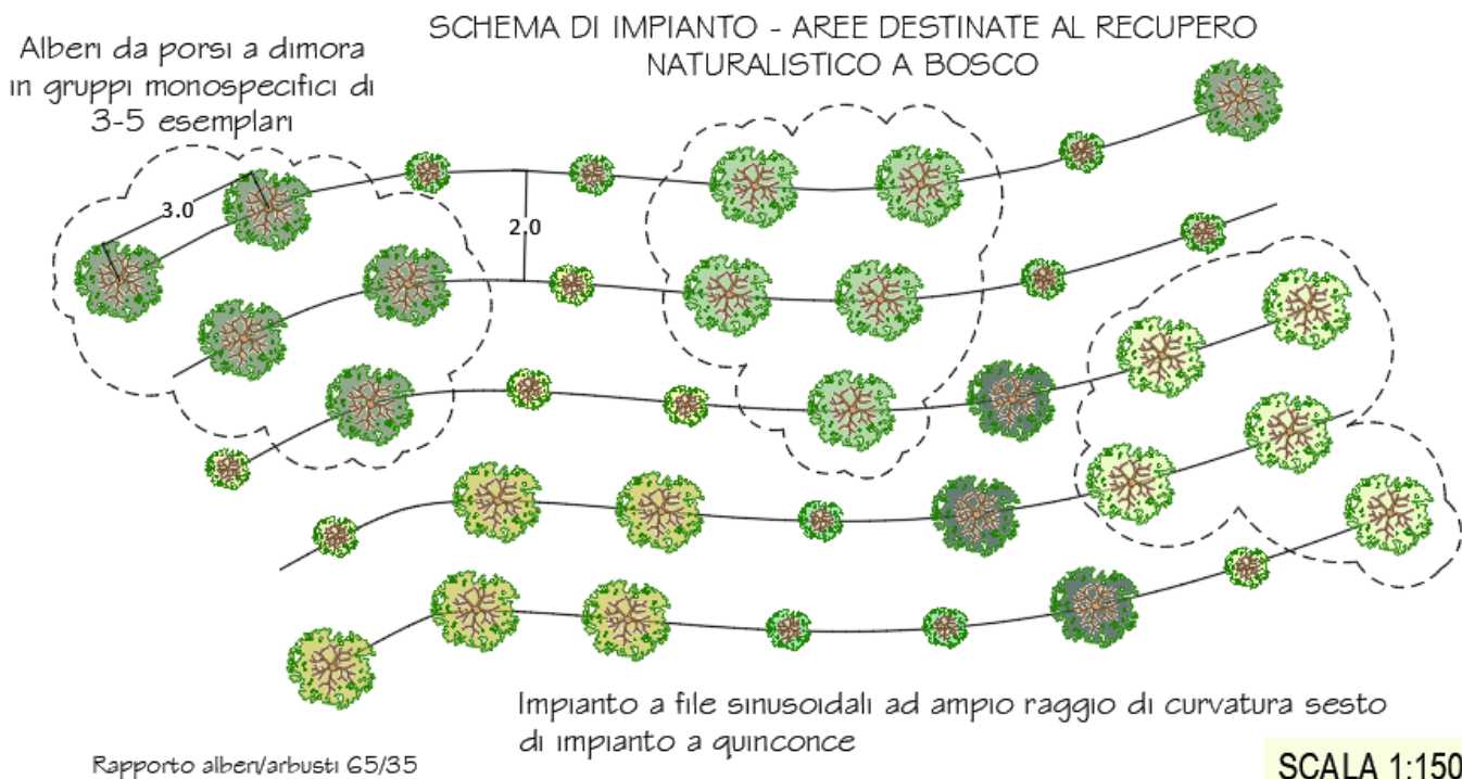
Figura 6. Schema di impianto per il recupero naturalistico a bosco (non in scala).
