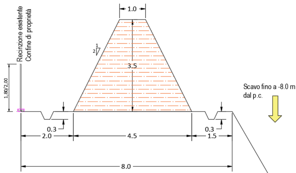
Figura 3. Tipologico della duna posta nell'area di rispetto
