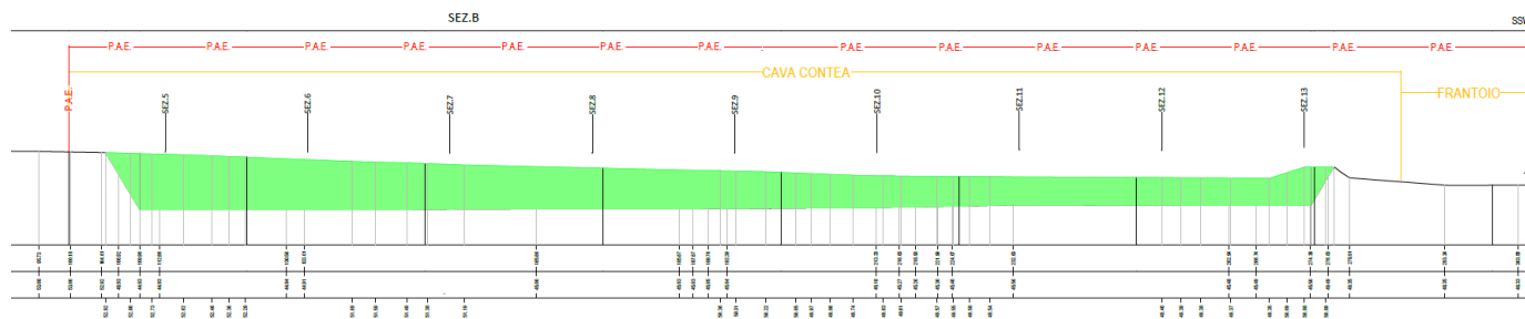
Figura 5. Sezione NNE-SSW esemplificativa degli interventi di recupero morfologico a piano ribassato con la porzione nord recuperata fino a piano campagna, la porzione meridionale recuperata con piano ribassato (max 4m da p.c. attuale) e la ricostruzione dell'argine di protezione della vasca esistente. In verde i riempimenti
