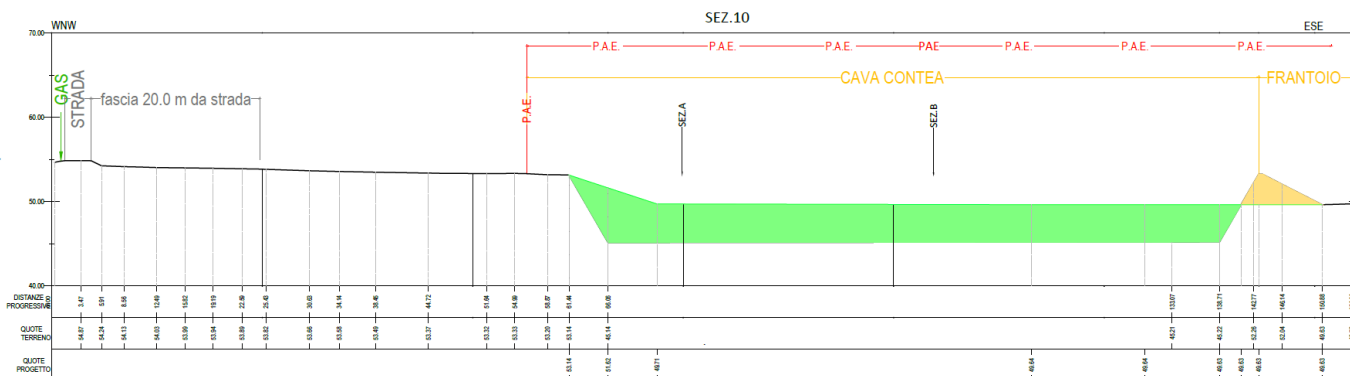
Figura 4. Sezione WNW-ESE esemplificativa degli interventi di recupero morfologico a piano ribassato. In verde i riempimenti ed in arancione le aree di modellazione morfologica in scavo
